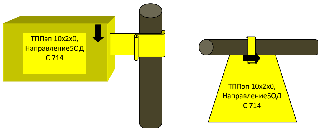
Рисунок 4 Пример маркировки кабелей
