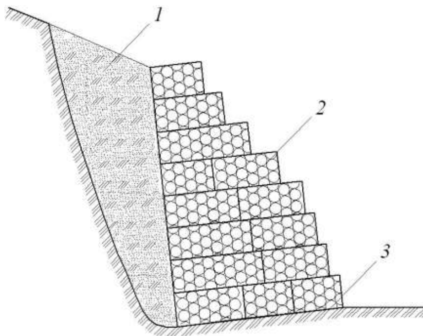
Рисунок 5 – Пример конструкции массивно-объемной стены со ступенчатой лицевой гранью на наклонном основании с обратной засыпкой
