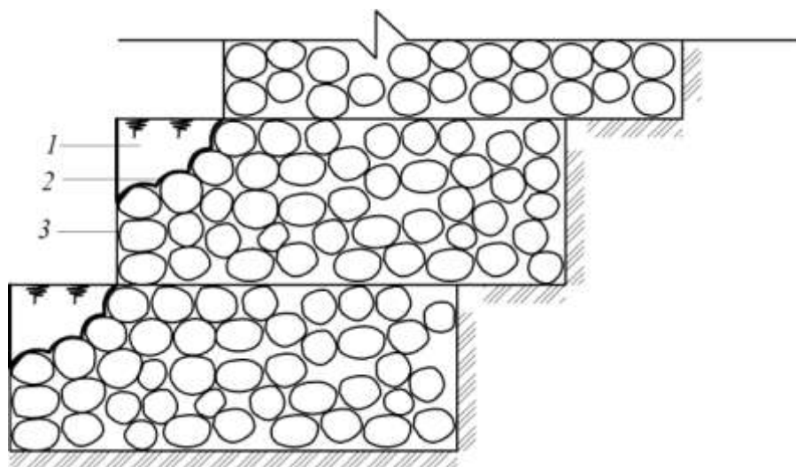
Рисунок 2 – Пример заполнения коробчатых габионных конструкций растительным грунтом
