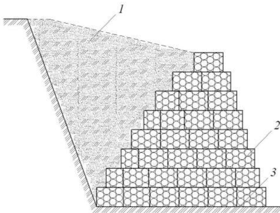
Рисунок 4 – Пример конструкции массивно-объемной стены со ступенчатой лицевой гранью на горизонтальном основании с обратной засыпкой
