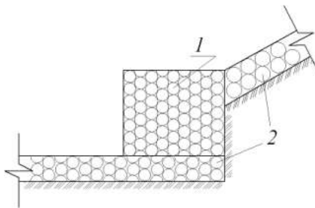
Рисунок 11 – Пример исполнения упорного элемента габионного сооружения
