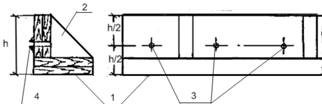
Рисунок 3 - Конструкция рабочего шва
